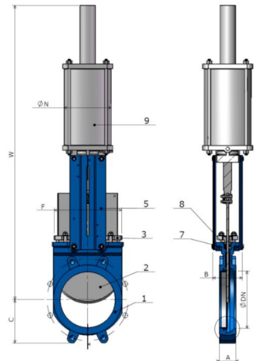
DN350
