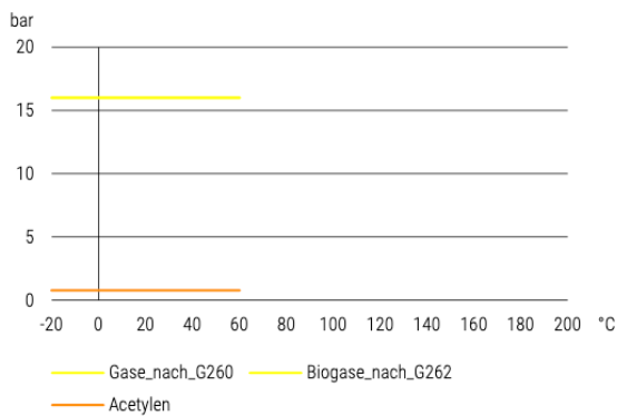
Druck-Temperatur-Diagramm pressure-temperature-diagram
