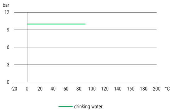
Druck-Temperatur-Diagramm pressure-temperature-diagram
